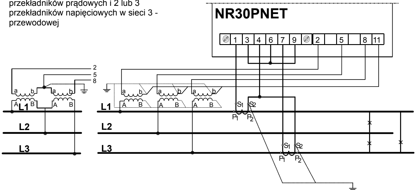
Rys.6. Podłączenia sygnałów wejściowych w sieci trójfazowej 3 – przewodowej
