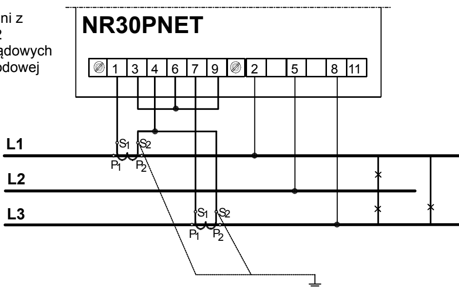
Rys.5. Podłączenia sygnałów wejściowych w sieci trójfazowej 4 – przewodowej
