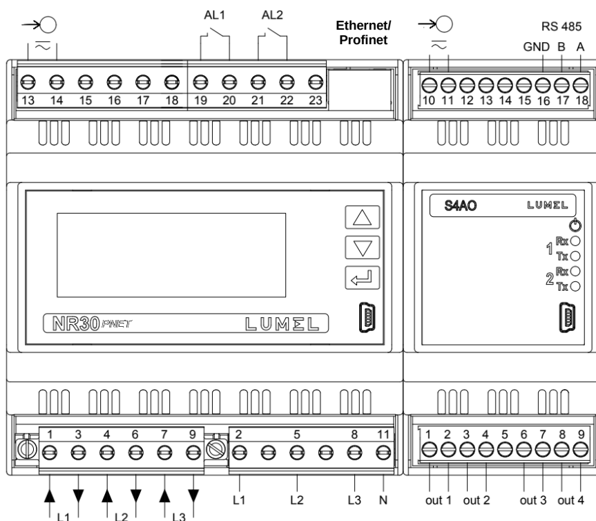
Rys.8. Podłączenie NR30PNET z S4AO interfejsem RS485
